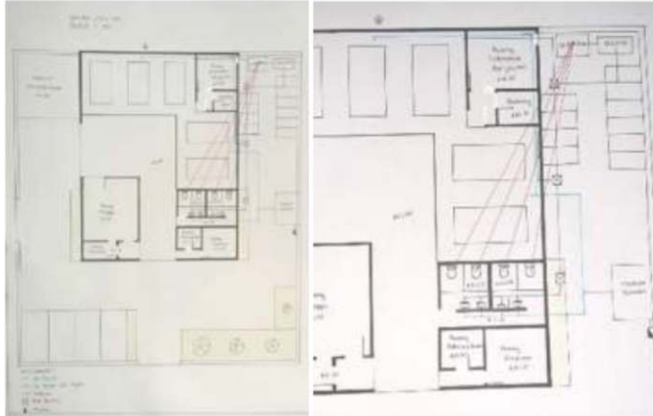
Gambar 7. Denah utilitas
