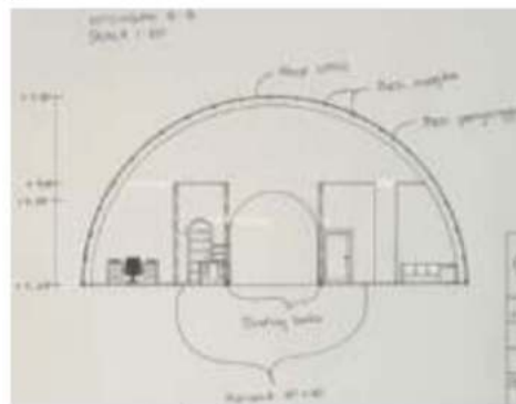
Gambar 8. Potongan B-B
