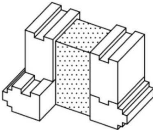
Gambar 6. Teknik penyambungan 3 lapis
