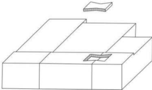
Gambar 5. Teknik penyambungan ekor burung pada batuan
