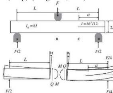
Gambar 9. Spesimen ENF dan sketsa analisis mekanika
