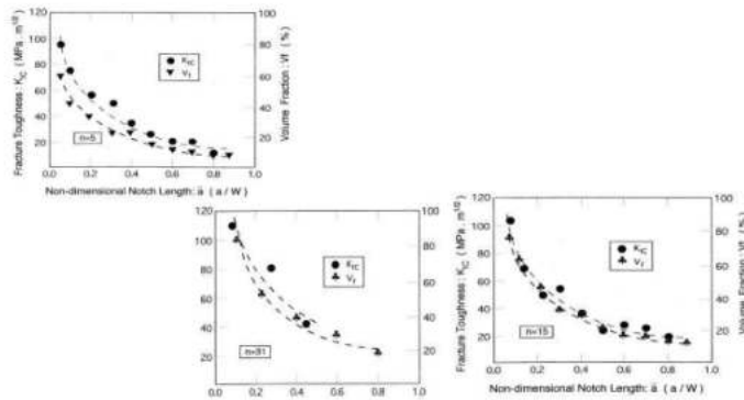
Gambar 8. Ketangguhan patah pada ketebalan bambu pada berbagai ketinggian Sumber: Sulastiningsih, 2013
