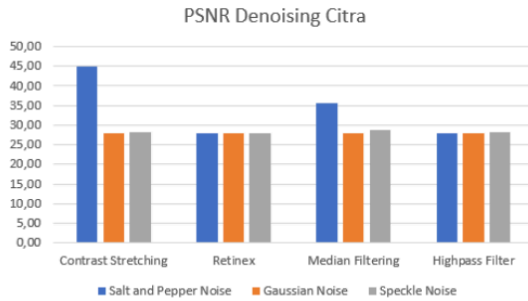
Gambar 5. Diagram Perbandingan PSNR
