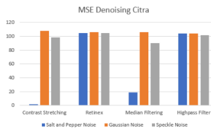
Gambar 4. Diagram Perbandingan MSE
