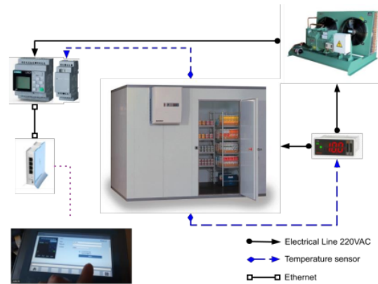
Gambar 1. Kontrol elektronik dan data logger ruang dingin menggunakan sensor suhu PT100
