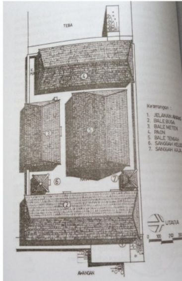
Gambar 9. Peruangan rumah tinggal standar di desa Pagringsingan Sumber: Runa, 2018:140
