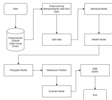
Gambar 1. Langkah-langkah pengujian kedua model
