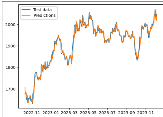
Gambar 2. Prediksi SARIMAX (ARIMA)
