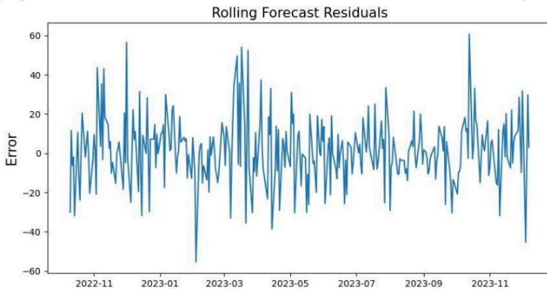
Gambar 6. Prediksi salah Arima
