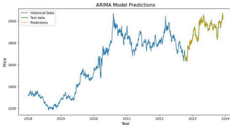
Gambar 4. Prediksi tahun 2024 Arima
