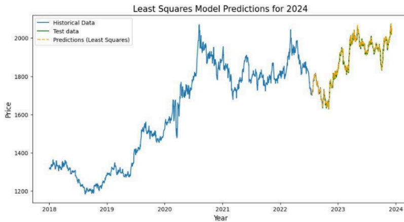
Gambar 5. Prediksi tahun 2024 Least Square
