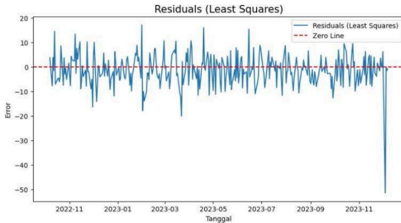
Gambar 7. Prediksi salah Least Square
