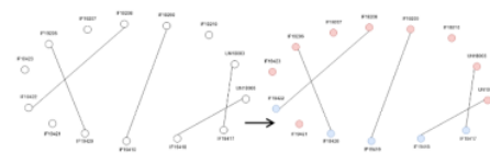
Gambar 8. Hasil pewarnaan graf dengan algoritma welch-powell
