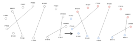
Gambar 9. Hasil pewarnaan graf dengan algoritma recursive largest first
